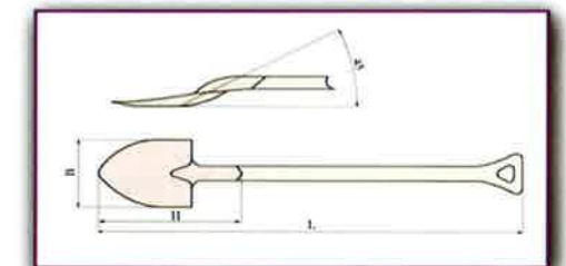
Shovel, round point Schaufel, Frankfurter Form, DIN 20121 Pala de Punta Redonda
