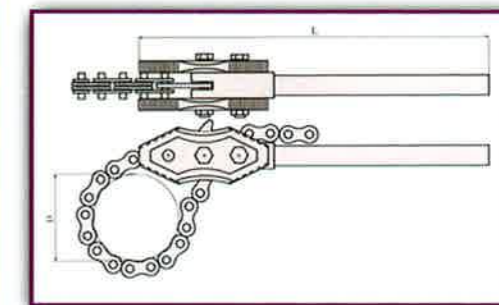
Chain pipe wrench Kettenrohrzange Llave Encadenadora de Tubos
