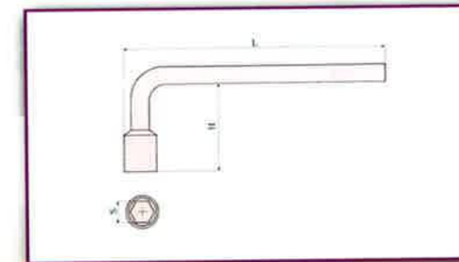
Socket wrench L-type, 6 point Steckschlüssel, gewinkelt, 6-kant Llave para Cubo, Tipo-L, 6 puntos
