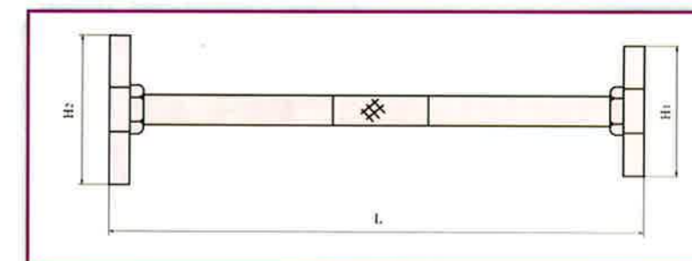
Multi-head bung wench Universalfasschlüssel Llave taponadora universal
