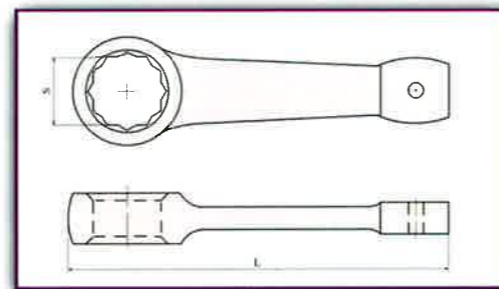
Striking box wrench 12 point Ringschlagschlüssel, 12-Kant, DIN 7444 Llave de Cajon de Golpe, 12 Puntos
