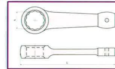
Striking box 12 point Ringschlagschlüssel, 12-kant, DIN 7444 Llave de Cajon de Golpe, 12 Puntos
