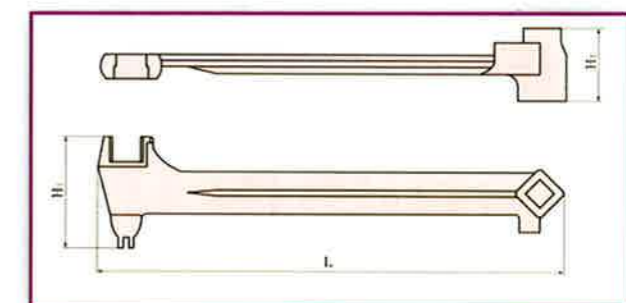
Multi-head bung wench Universalfasschlüssel Llave taponadora universal
