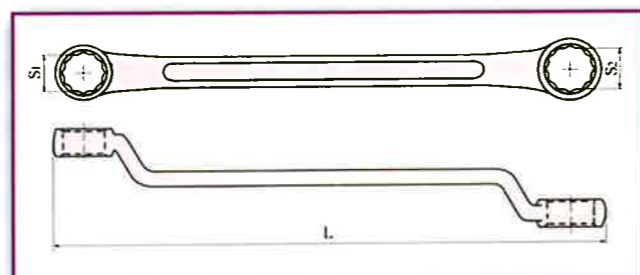
Double end box wrench offset Doppelringsschlüssel gekröpft, DIN 838 Llave de Cajon Doble tipo acodado
