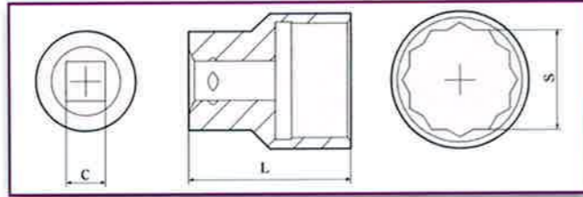
Sockets Steckschlüsseinsätze Cubos
