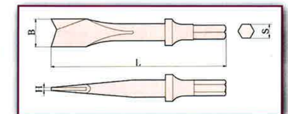
Chisel pneumatic Pneumatischer meißel Buril neumatico
