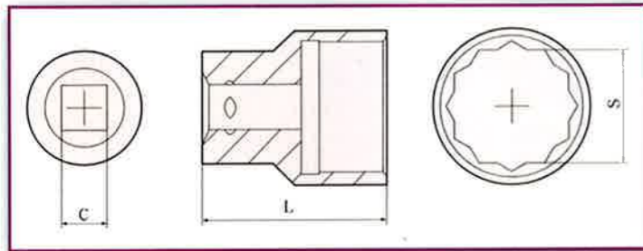
Sockets Steckschlüsseinsätze Cubos
