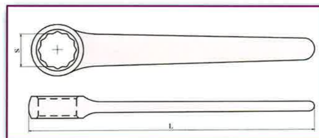
Single end box wrench Einfachringschlüssel, DIN 3111 Llave de Cajon Sencilla
