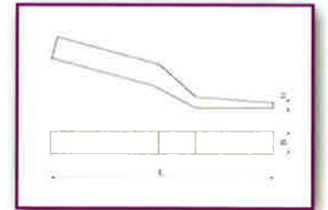
Caulking tool, flat edge, offset Stemmwerkzeug, Kante stumpf, gekröpft Herramienta de Rematar
