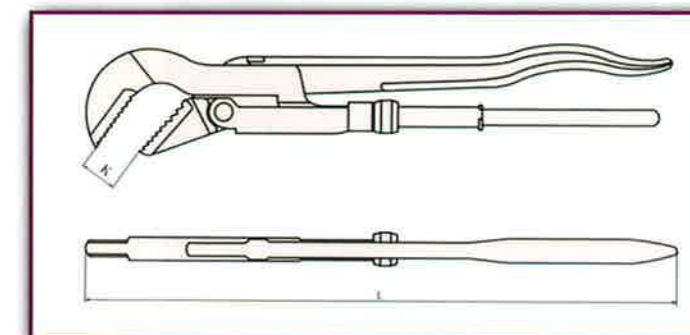
Pliers, Swedish Eckrohrzange Pinza Sueca
