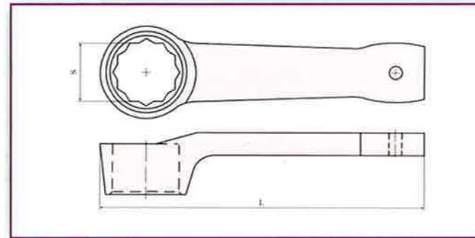
Double hex ring spanner- offset - flogging Ringschlagschlüssel, gekröpft Llave de cajon de Golpe, 12 puntos
