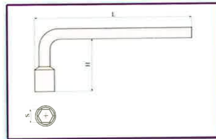
Socket wrench L-type, 6 point Steckschlüssel, gewinkelt, 6-kant Llave para Cubo, Tipo-L, 6 puntos
