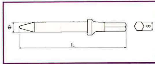
Chisel pneumatic Pneumatischer meißel Buril neumatico
