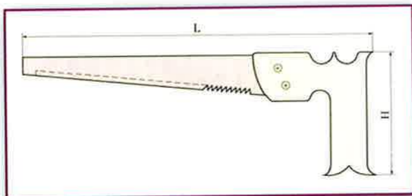
Hand saw Handsäge Serrucho de Mano
