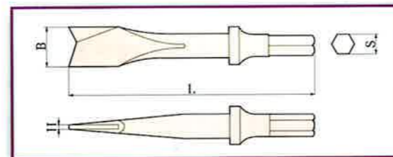
Chisel pneumatic Pneumatischer meißel Buril neumatico
