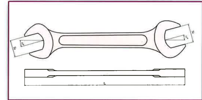
Double open end wrench Doppelmaulschl, DIN 895 Liave de Boca Doble
