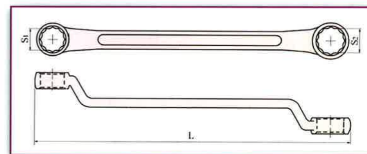
Double end box wrench offset Doppelringschlüssel gekröpft, DIN 838 Llave de Cajon Doble tipo acodado
