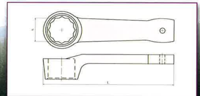
Double hex ring spanner- offset - flogging Ringschlagschlüssel, gekröpft Llave de cajon de Golpe, 12 puntos
