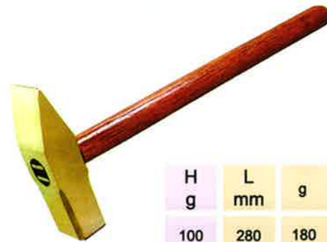
Hammer, cross pein engineer's Schlosserhammer, DIN 1041 Martillo de Ingeniero de Golpe Cruzado
