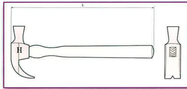
Hammer, claw Klauenhammer Martillo con Garra
