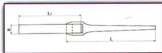
Wrench, Belt Pipe Kettenrohrlicht-schlüssel Llave, luz de cadena de la pipa
